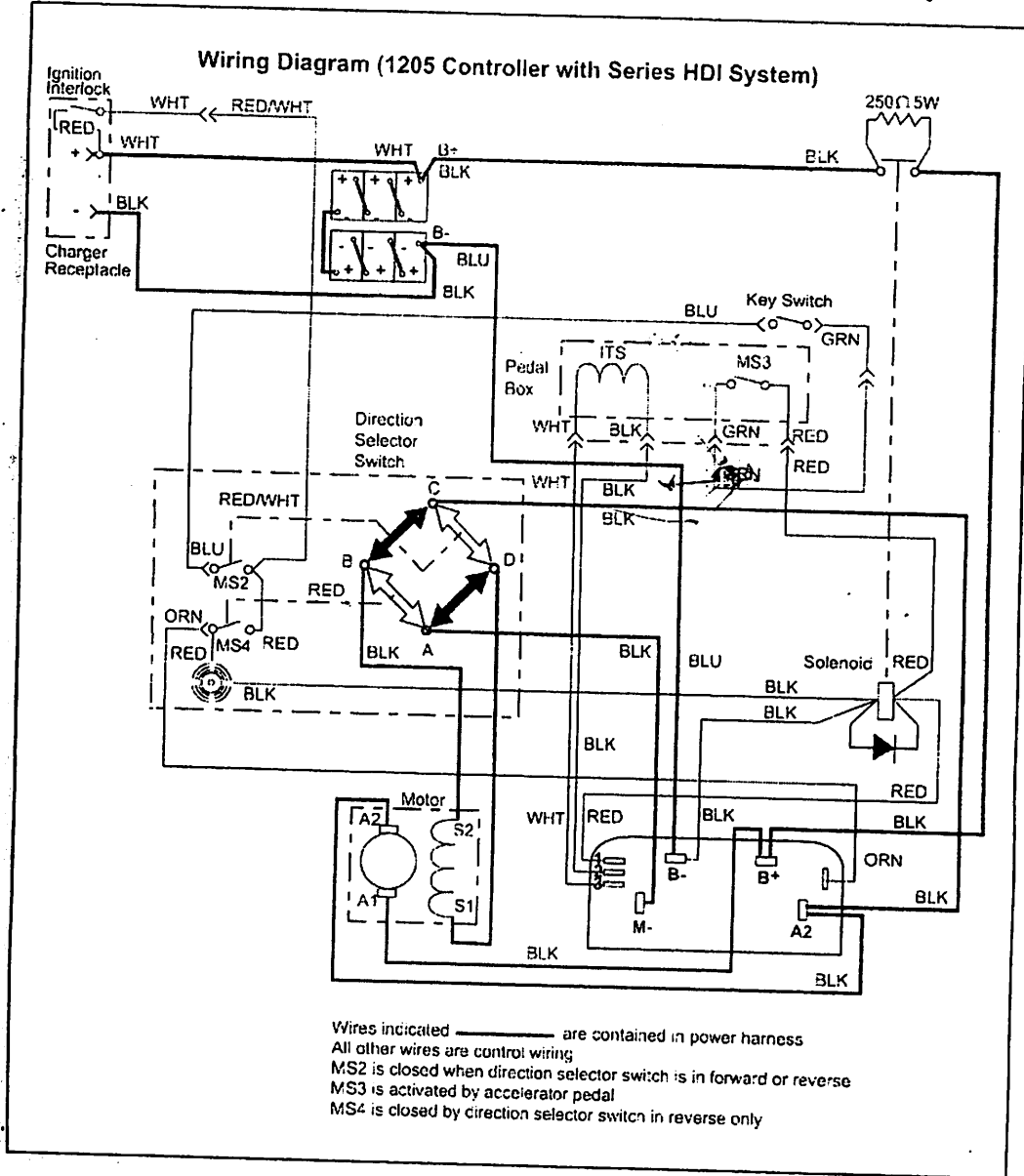
Fig. 18 Wiring Diagram
