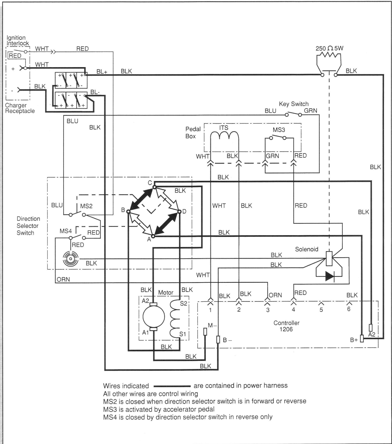
Fig. 19 Wiring Diagram
